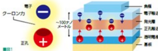
■図1 エキシトンの構造と、電子と正孔がペアになり、普通より高いエネルギーを持っている状態。 ■図2 有機EL素子の構造
