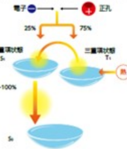
■図3 発光原理熱活性化遅延蛍光(TADF)
