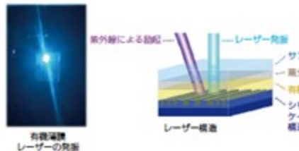
■図5 有機薄膜レーザーの光の構造
