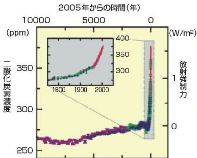
図3 大気中の二酸化炭素濃度の推移
