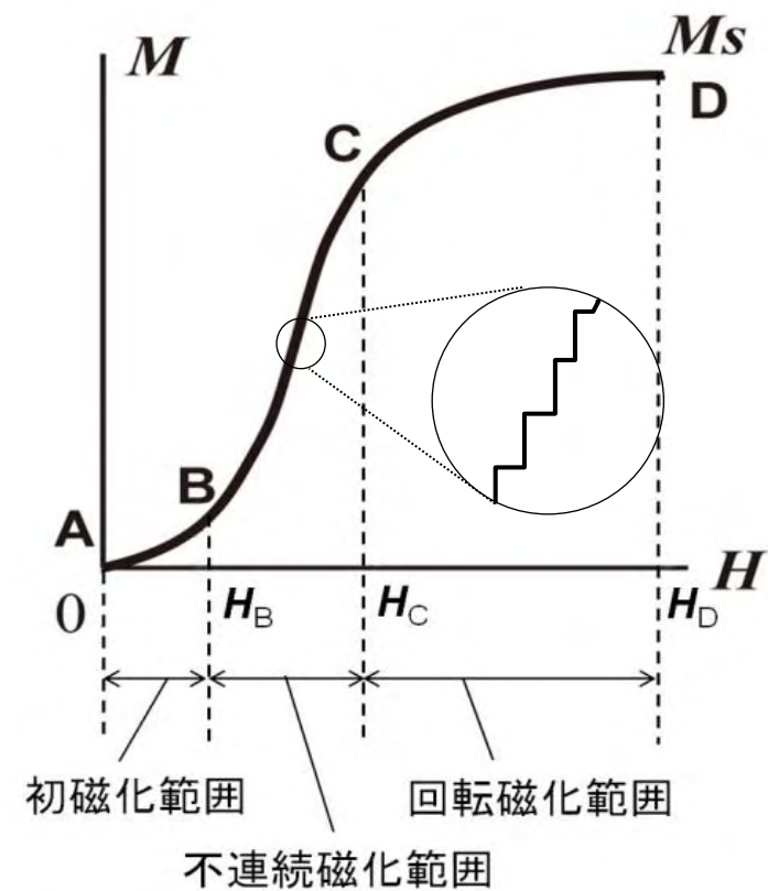
図5.6 初磁化曲線
