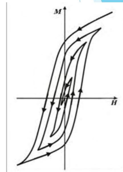
図5.8 交流消磁の消磁過程
