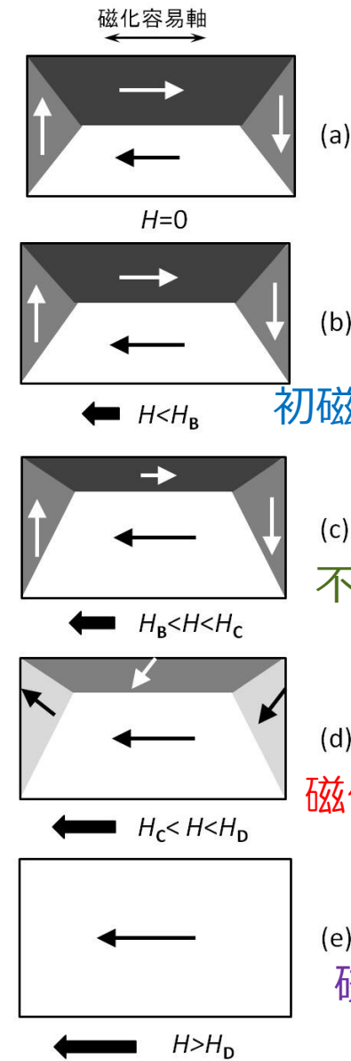
図5.7 初磁化曲線の磁壁移動・磁化回転による説明
