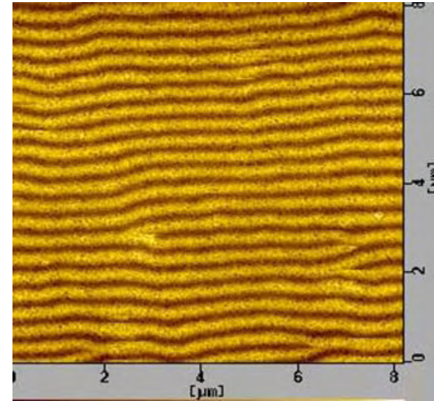
図4.10 磁気力顕微鏡(MFM)で見た縞状磁区の像
