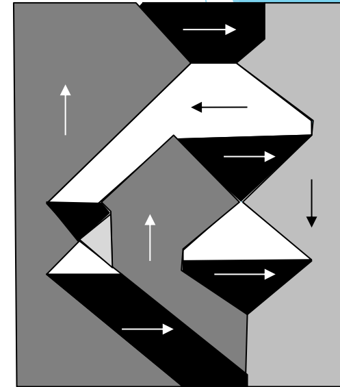
図4.2 磁化前の磁性体の磁区構造の模式図
