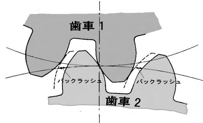
図5.5 歯車もヒステリシスをもつ
