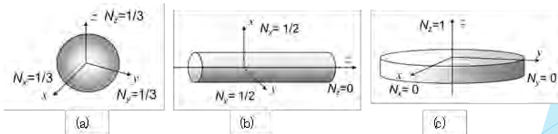
図4.6 反磁界係数は磁性体の形と向きで異なる。
