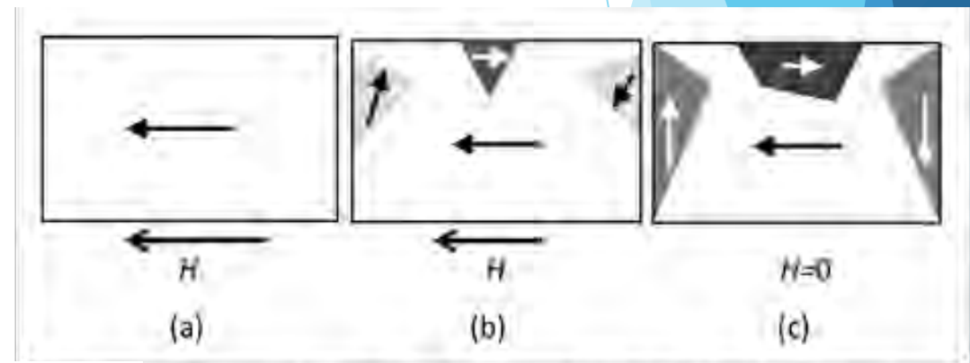
図5.16 磁気飽和状態から磁界を減らしていくと、さまざまな磁化方向の磁区が核発生し、成長するが、もとの状態には戻れない。
