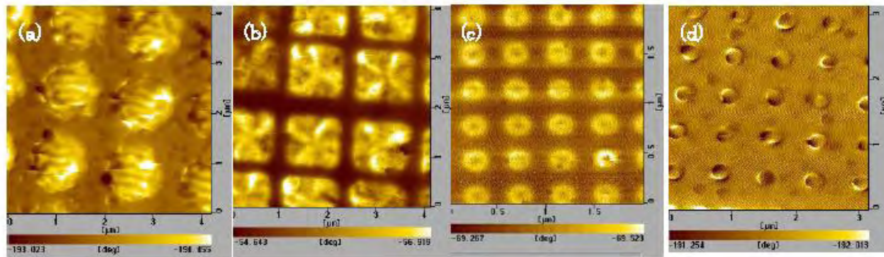
図 4.14 微細ドットの磁気構造 (a) 渦状磁区(Co 円形ドット 1.2\mu\text{m}\phi ), (b) 環流磁区(パーマロイ正方形ドット 1.2\mu\text{m} ), (c) ボルテックス(パーマロイ円形ドット 300\text{nm}\phi ), (d) 単磁区(Co 円形ドット 100\text{nm}\phi )
