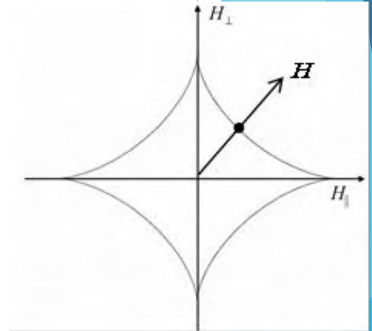
図5.17 磁化反転の臨界磁界曲線
