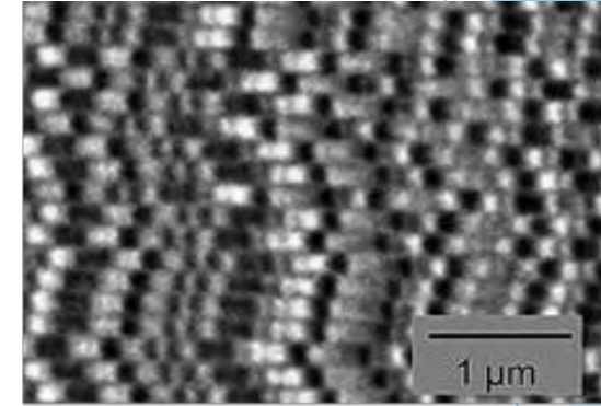
図5.1 垂直磁気記録された記録磁区のMFM像（中央大学二本先生による）
