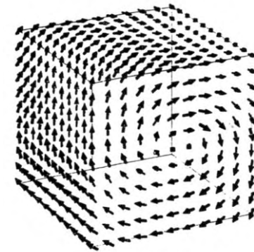
図4.13 ボルテックス構造
