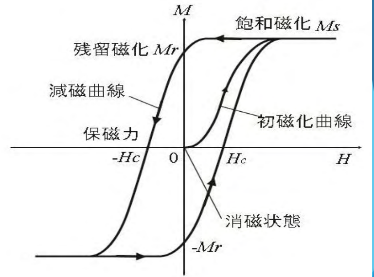
図5.3 強磁性体の典型的な磁化曲線
