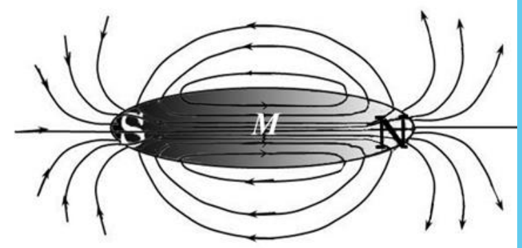
図4.4 磁束線は磁化と連続
