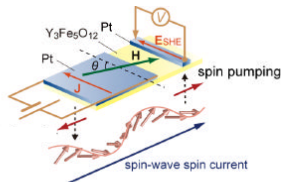
図1 誘電体スピン流伝送の概念図
